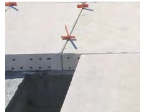
Fig. 6: Separación de la Junta.
