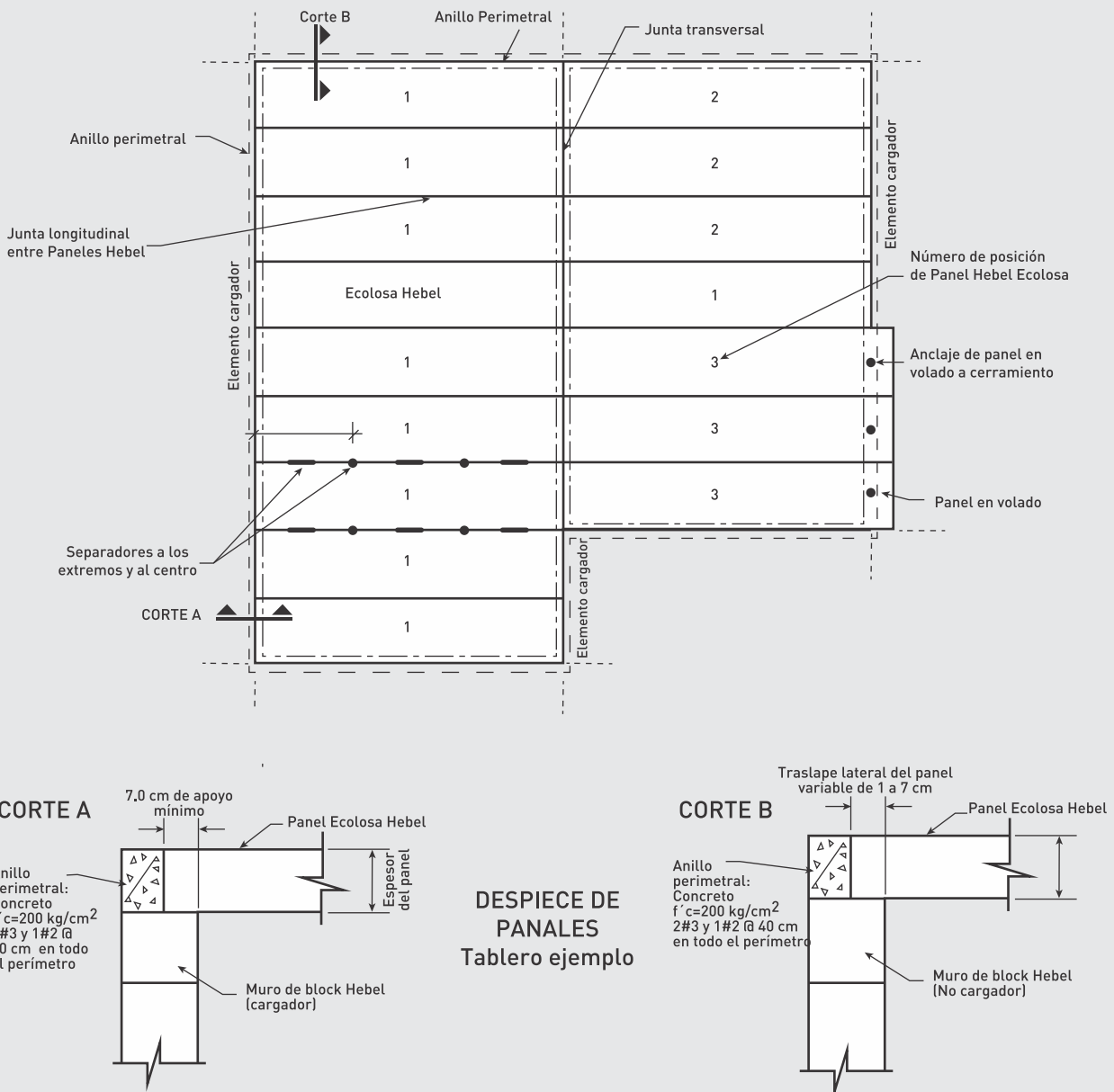
Fig. 10: Tablero tipo de apoyo de paneles sobre mampostería.
